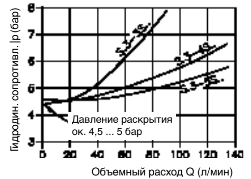
Циркул. сопротивление при разгруженной расходомерной диафрагме
