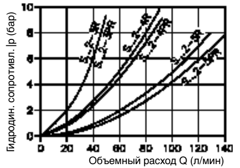
Циркул. сопротивление при разгруженной расходомерной диафрагме
