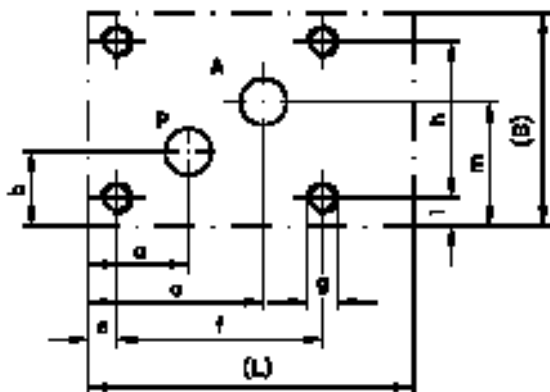
Схема отверстий в опорной плите (вид сверху)
