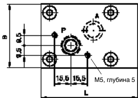
Схема отверстий в опорной плите (вид сверху)
