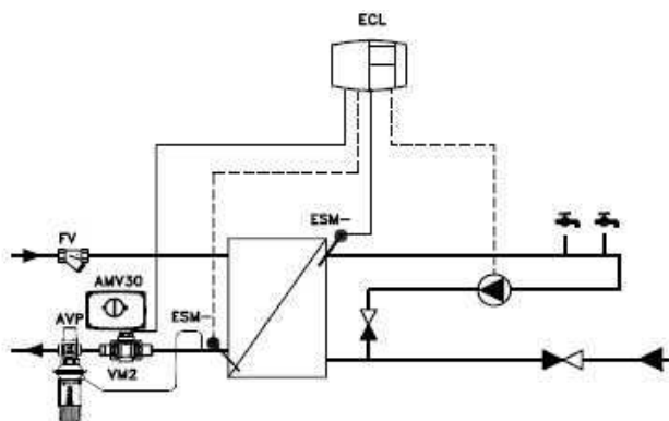
Рис. 2. Пример применения клапанов в системе горячего водоснабжения с водонагревателем.
